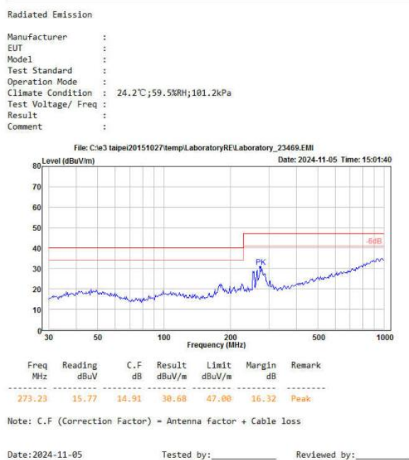
图 5-6 辐射测试水平方向
