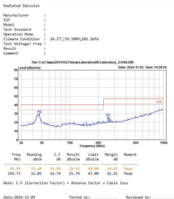
图 5-7 辐射测试垂直方向
