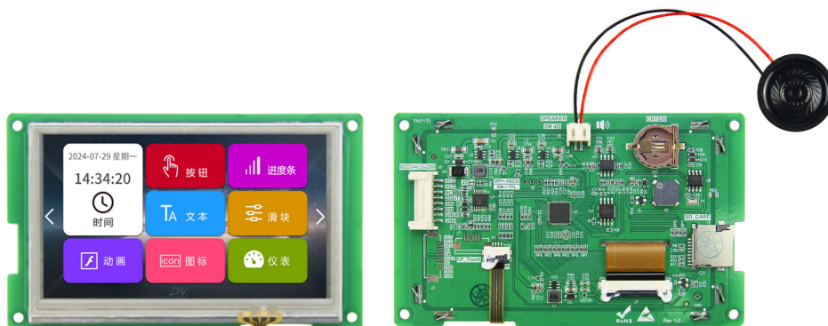
图 1-1 4.3 寸电阻触摸参考图
