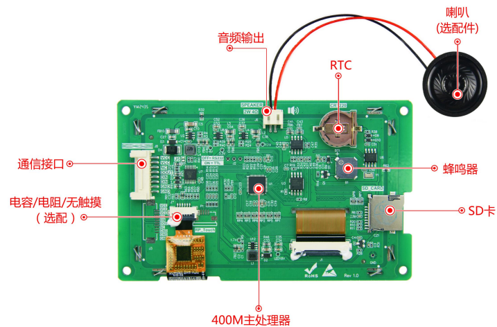
图 1-4 硬件配置图
