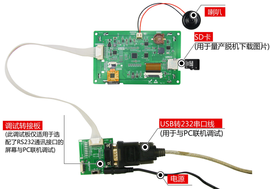
图 1-5 调试工具图
